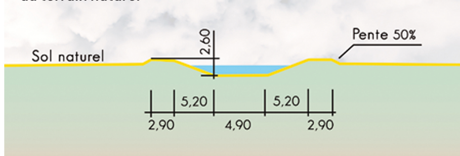
Profil en travers type du Canal suivant les courbes de niveau du terrain naturel
